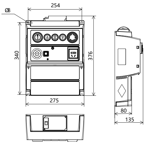
图 3 安装尺寸示意图（单位：mm）
